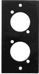
RSP-12D FRONTAL 1 SEGMENTO 2 CONECTOR SERIE D
