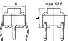
SW0232E PULSADOR TACTO 6x6 mm 12V 50 mA 5 PIN L : 8.00 mm
