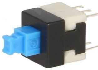
SW0214 CONMUTADOR 2 CIR DPDT 0.1A 30 VDC 8x8 mm
