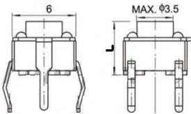
SW0232B PULSADOR TACTO 6x6 mm 12V 50 mA 5 PIN L : 7.00 mm
