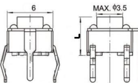
SW0232F PULSADOR TACTO 6x6 mm 12V 50 mA 5 PIN L : 12.50 mm
