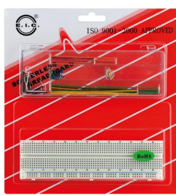
Código: BP008 Fabricante: EIC Ref. Fabricante: EIC101J Numero Puntos : 730 Puentes
