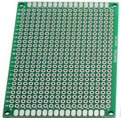
PCB DOBLE CARA ESTAÑADA 50 X 40 R 2.54 mm PCB203
