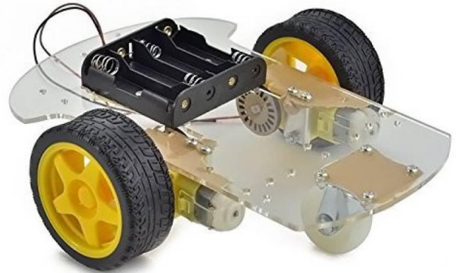
RT9005 KIT DE CHASIS DE COCHE 2 WD CON ENCODERS Y MOTORES
