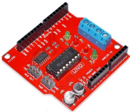
MD0224 MODULO CONTROL L298N
