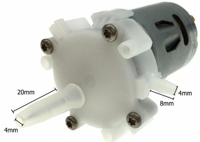
MT0103 BOMBA AGUA SUMERGIBLE JT-DC3W 3-5VDC 0.18 A 100L/H 35 CM
