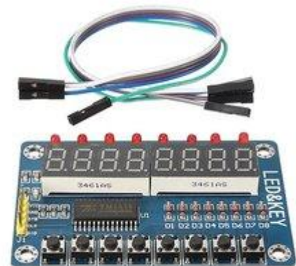
TM1638 MODULO DISPLAY 8 BITS CON TECLADO 8 PULSADORES
