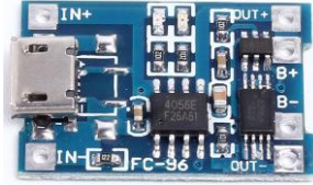
MD9084 Micro USB Módulo de carga Li-ION 3V7 1 A Protección de Carga, Sobrecorriente y Descarga
