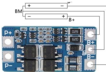
MD9129 2S10A Li-ion 18650 Lithium Batería Placa de protección del cargador 8.4V Sobrecorriente Sobrecarga. Protección contra descarga excesiva
