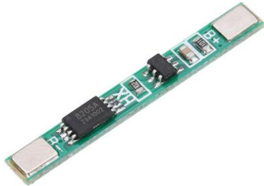
MD9196 1S03A Li-ion 18650 Lithium Batería Placa de protección del cargador 3.7V Sobrecorriente Sobrecarga Protección contra descarga excesiva
