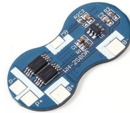
WH-2S80A 2S Li-ion 18650 Lithium Batería Placa de protección del cargador 7.4V Sobrecorriente Sobrecarga Protección contra descarga excesiva
