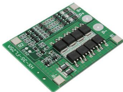
3S 25A PCB Placa de Protección de la Batería de Litio Li-ion 18650 BMS con Función de Equilibrio 12.6V 25A
