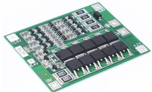
MD9128 4S 40A PCB Placa de Protección de la Batería de Litio Li-ion 18650 BMS con Función de Equilibrio 16.8V 40A
