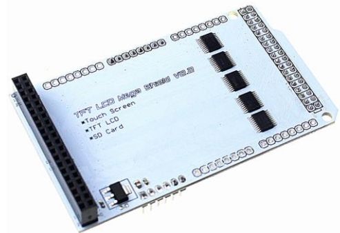
MD9096 MODULO SHIELD MEGA - PANTALLA TACTIL TFT320QVT
