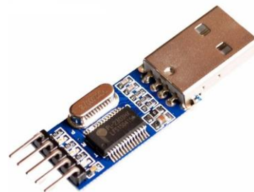
MD9165 MODULO USB A TTL PL2303HX SMT32
