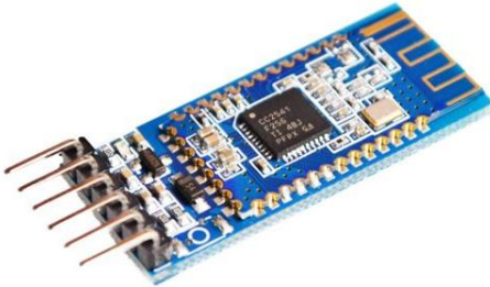
MD9187 MODULO BLUETOOTH HC-08
