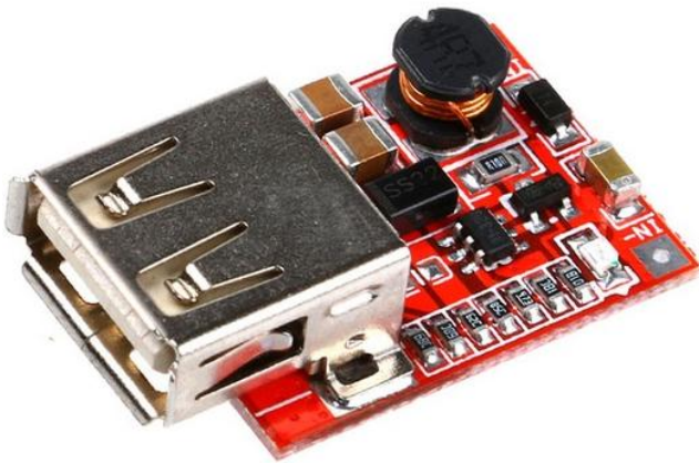
MD9094 Módulo STEP UP Li-ION 3V7 A 5V 1 A Proteccion Sobrecorriente y Descarga
