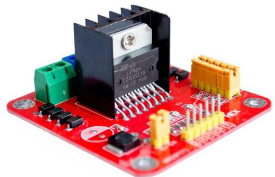
MD9031 MODULO CONTROL MOTOR DUAL PUENTE H L298N
