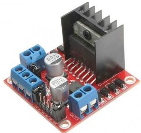
MD9031 MODULO CONTROL MOTOR DUAL PUENTE H L298N
