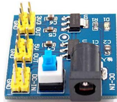
MD9114 MODULO ALIMENTACION 3.3- 5 - 12 VDC SALIDA 12 VCC ENTRADA
